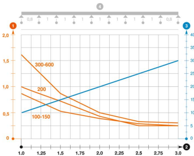
Diagrama de cargas do caminho de cabos GR-Magic do tipo GRM 105
