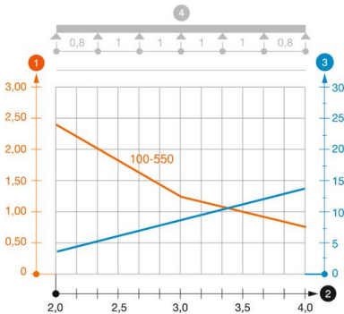
Diagrama de cargas do caminho de cabos em chapa SKSU 110
