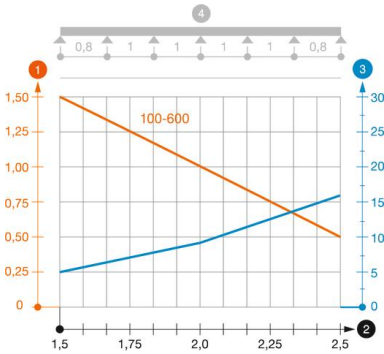
Diagrama de cargas do caminho de cabos do tipo MKS 60
